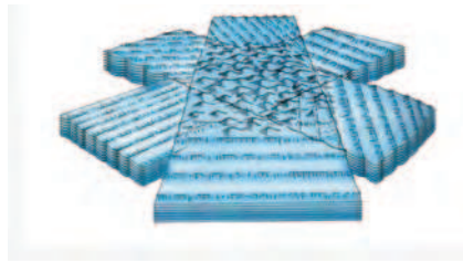
Les vagues internes à l'interface entre deux couches d'eau de densités différentes. L'une est dense (celle du bas), l'autre est moins dense (celle du haut). (Oceanography, Gross, p. 204)
