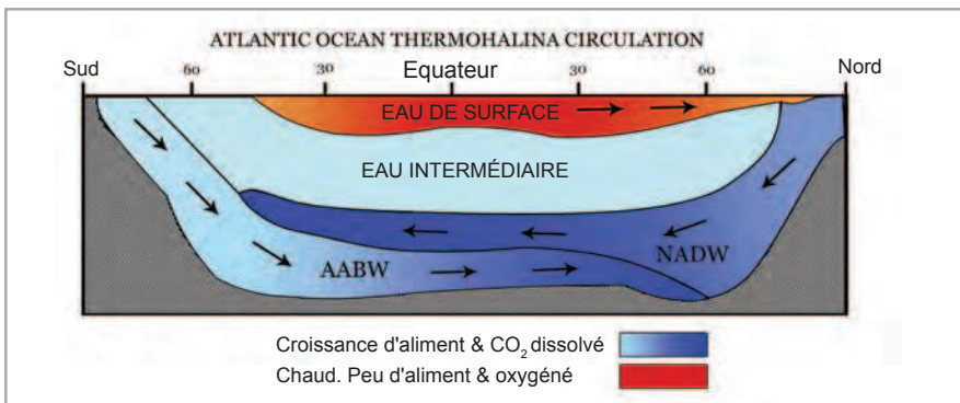
Les masses d'eau importantes dans l'océan profond se différencient par leur température et leur salinité. Ces propriétés déterminent leurs densités relatives, qui à son tour conduit la circulation thermo haline profonde des océans.. NADW = North Atlantic Deep Water. AABW = Antarctic Bottom Water. Mise à jour de la courtoisie figure de Dr. Steve Hovan, Indiana University of Pennsylvania.
